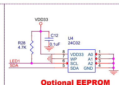
Optional EEPROM
